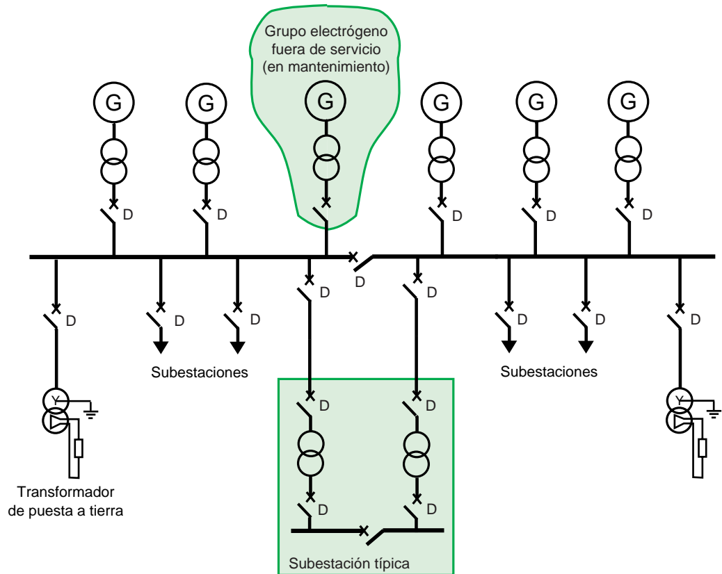
Fig. 5: Emplazamiento industrial sin conexión a la red general. Todos los interruptores automáticos identificados como «D» está normalmente cerrados.
