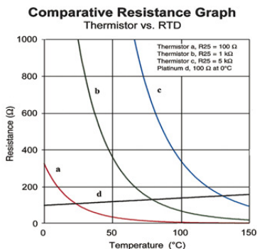
Curvas de termistores comparadas con un RTD
